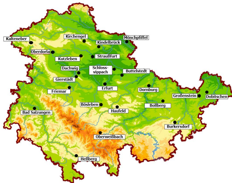
Abb. 1: Monatsmittel der Lufttemperatur und des Niederschlages für den März 2023 und deren Abweichungen von den vieljährigen Durchschnittswerten ausgewählter Wetterstationen
