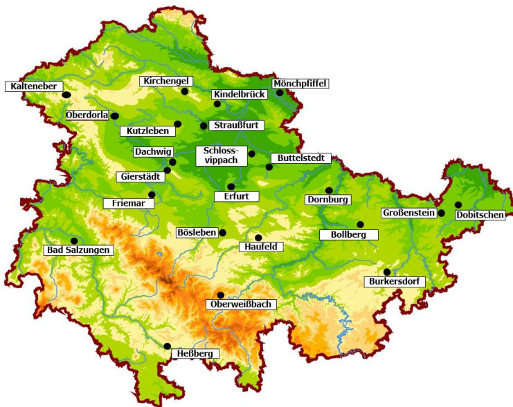
Abb. 1: Monatsmittel der Lufttemperatur und des Niederschlages für den Juli 2022 und deren Abweichungen von den vieljährigen Durchschnittswerten ausgewählter Wetterstationen
