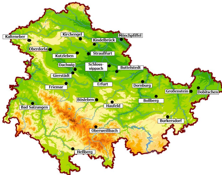
Abb. 1: Monatsmittel der Lufttemperatur und des Niederschlages für den April 2023 und deren Abweichungen von den vieljährigen Durchschnittswerten ausgewählter Wetterstationen
